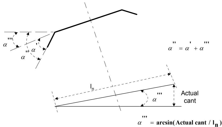
그림 12. 최고속도에서 Sloping Part of Bow의 각도
