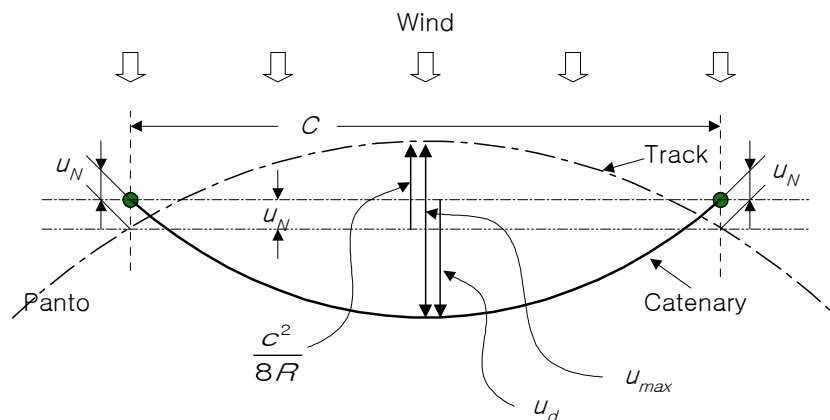
그림 19. 바람이 선로 내측으로 부는 경우 Catenary 변위
