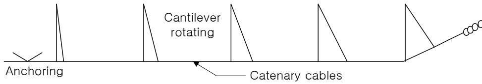
그림 15. 온도변화에 따른 캔티레버의 회전량 누증
