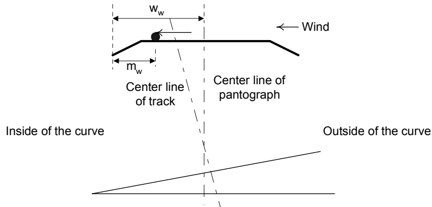
그림 4. 최고속도 열차주행, 곡선외측으로부터 최대풍압이 작용시 M_w
