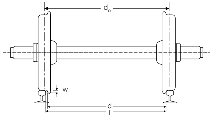
그림 7. 차륜 중심점사이 거리
