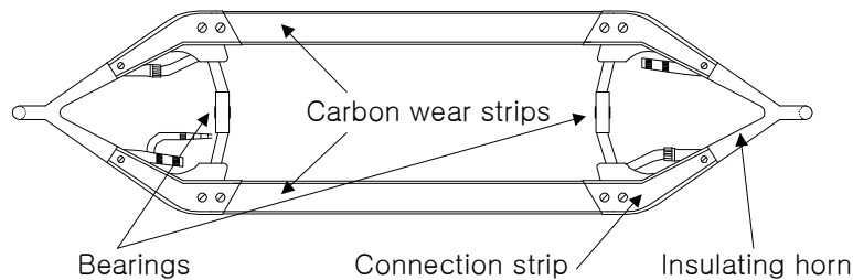
그림 8. 팬터그래프 Bow [GPU 25kV] (Top View)
