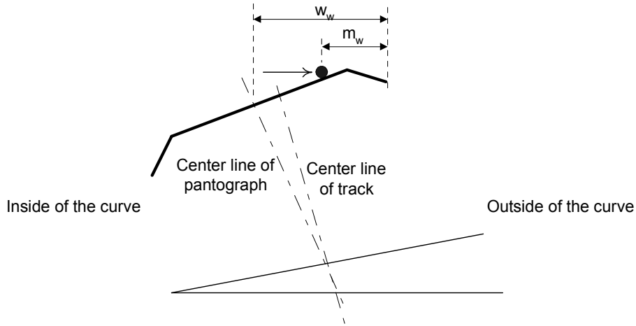
그림 3. 열차정지상태에서 전주 반대측에서의 M_w
