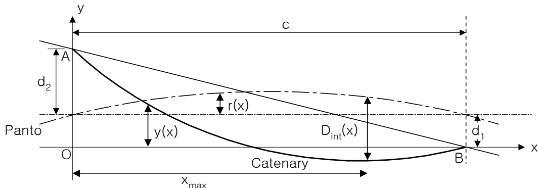
그림 22. 바람이 곡선 내측으로 부는 경우 Catenary 변위
