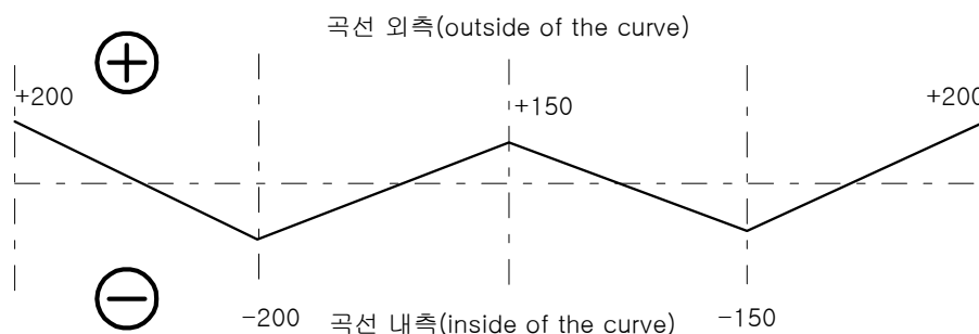
그림 14. 편위 부호 표기 원칙
