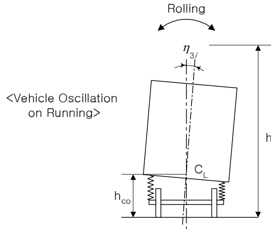
그림 13. 차량주행시 횡운동(Rolling)
