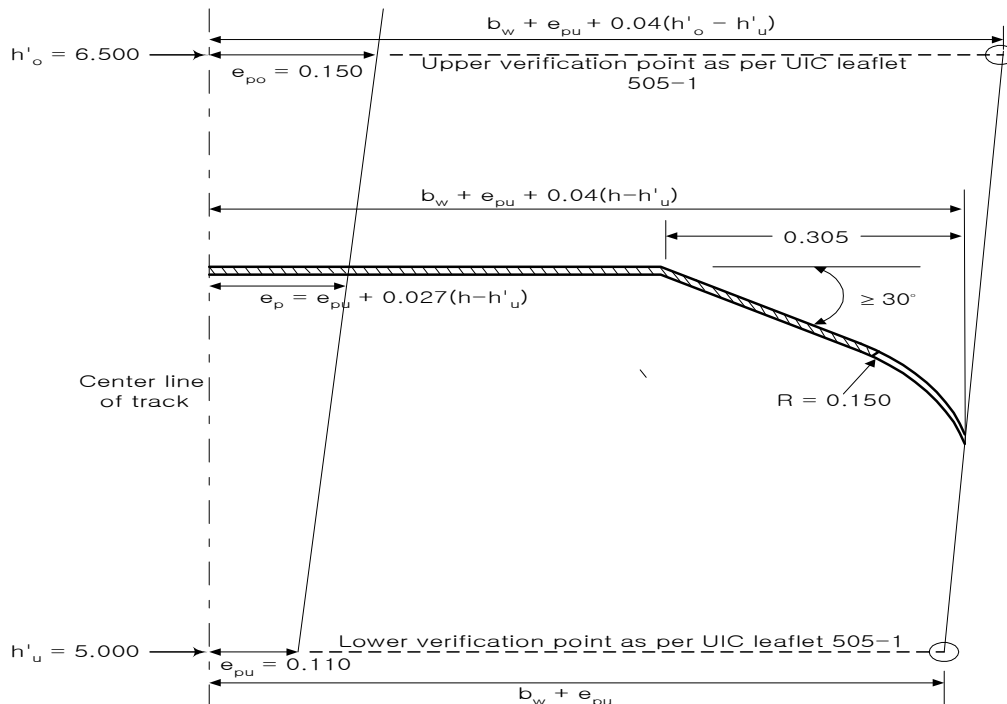
그림 10. Reference Outline for Pantograph
