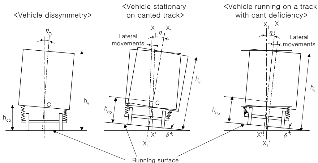
그림 6. 캔트/캔트부족량에 의한 영향
