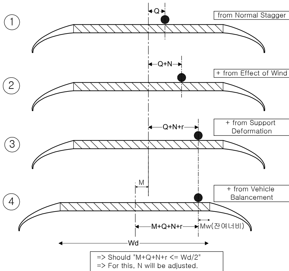
그림 2. 팬터그래프와 전차선의 횡적 위치 상호관계
