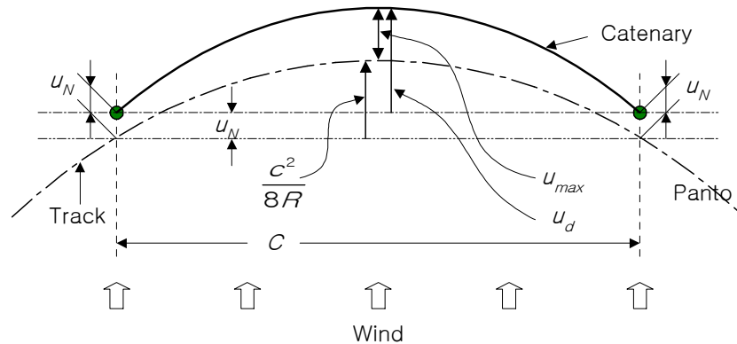
그림 20. 바람이 선로 외측으로 부는 경우 Catenary 변위
