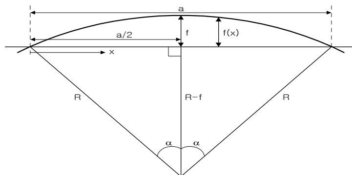
그림 18. 곡선선로에서의 기하학적 관계
