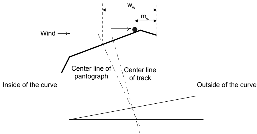
그림 5. 열차정지상태, 곡선내측으로부터 최대풍압이 작용시 M_w
