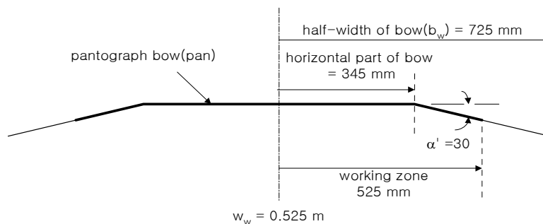
그림 9. Pantograph Working Zone
